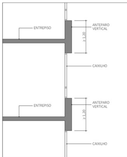
Figura C2 – Modelo de compartimentação com anteparo vertical.
