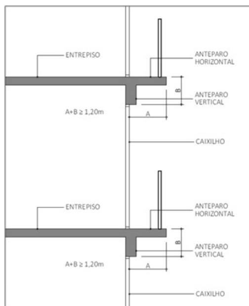
Figura C5 – Modelo de compartimentação com somatório de anteparos.
