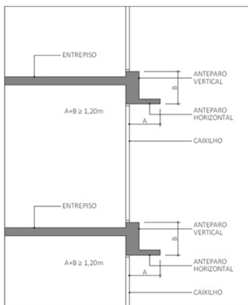
Figura C4 – Modelo de compartimentação com somatório de anteparos.
