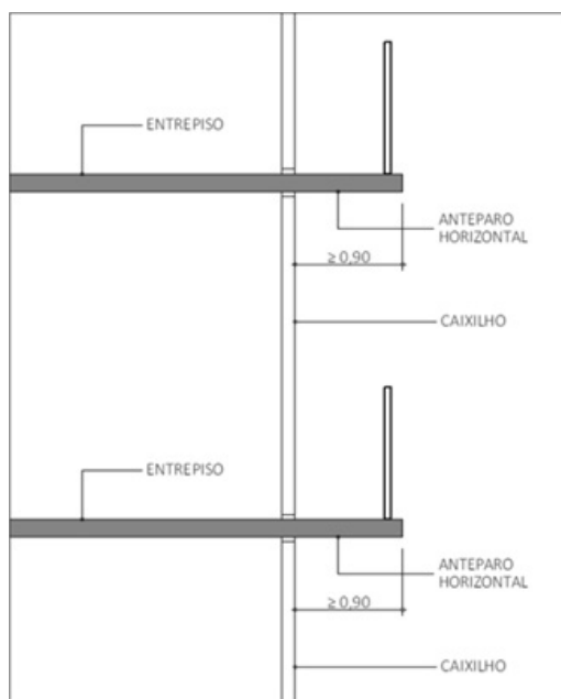
Figura C3 – Modelo de compartimentação com anteparo horizontal.
