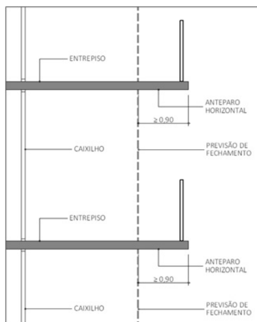
Figura C7 – Modelo de fechamento com vidro.
