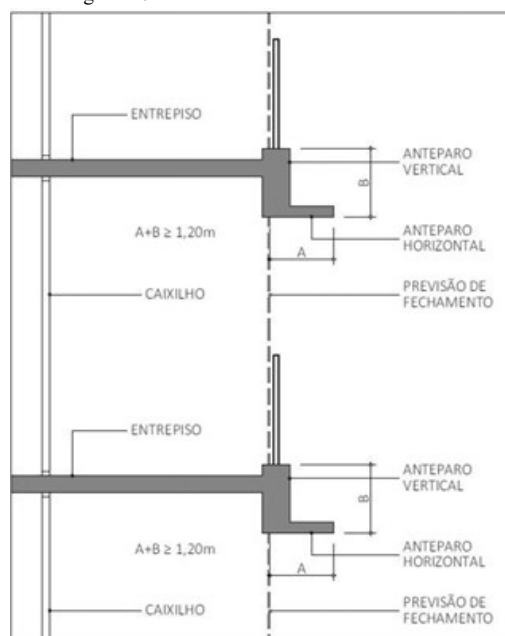
Figura C8 – Modelo de fechamento com vidro.
