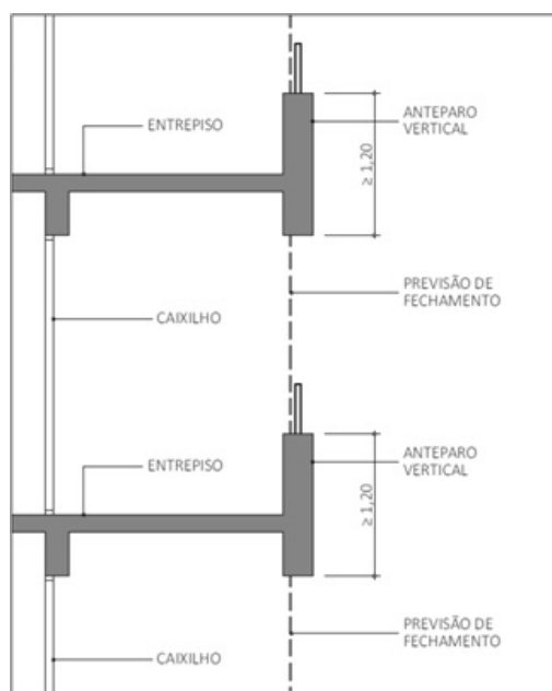
Figura C6 – Modelo de fechamento com vidro.
