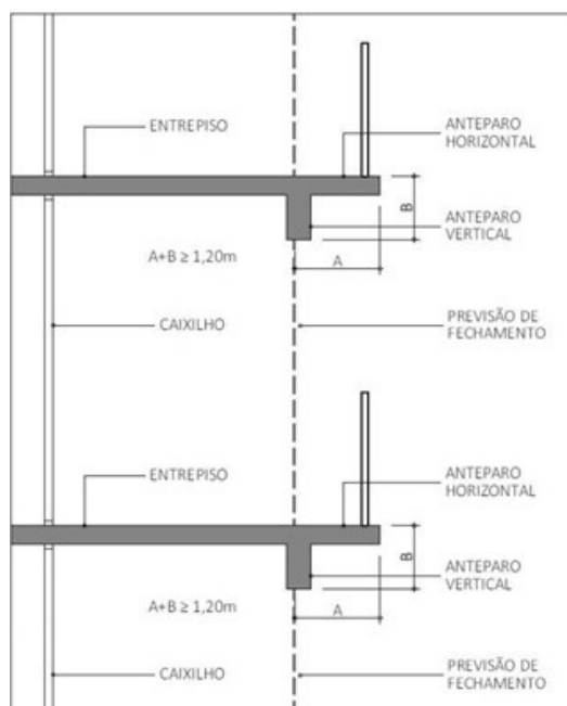
Figura C9 – Modelo de fechamento com vidro.
