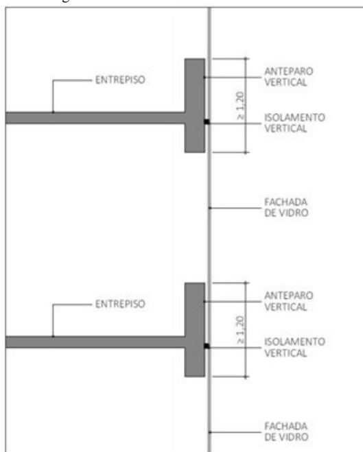
Figura C10 – Modelo de compartimentação com fachada envidraçada.
