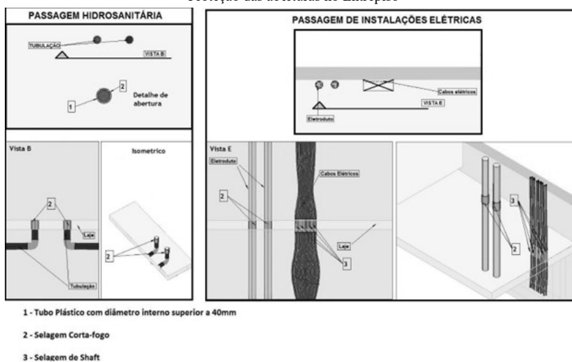
Figura D1 – Prumadas de instalações de serviços.
