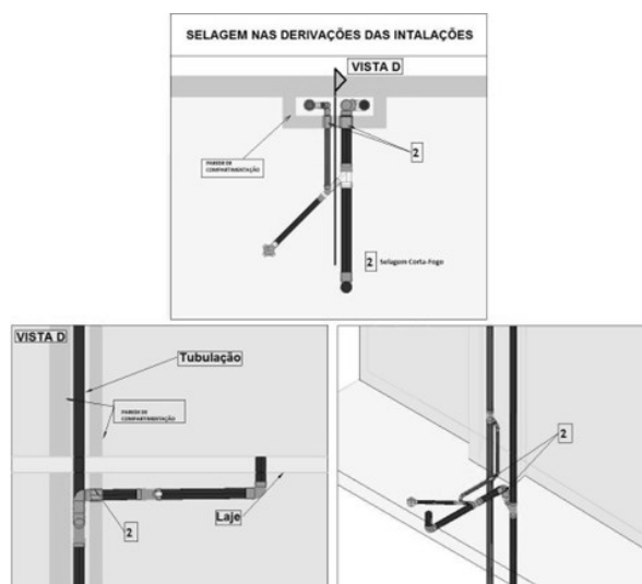
Figura D3 – Selagem nas derivações das instalações.
