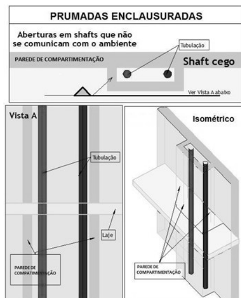
Figura D2 – Prumadas Enclausuradas.
