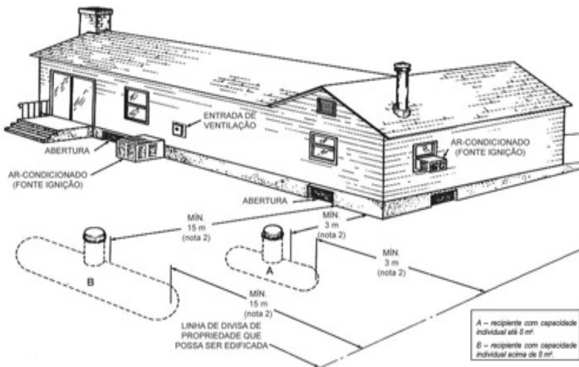
Figura 07: Instalação de recipientes estacionários enterrados
