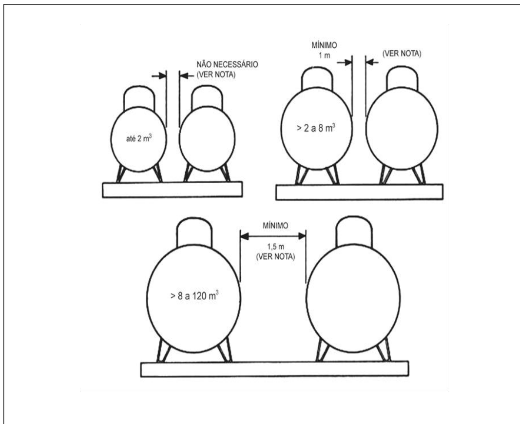
Figura 08: Distâncias entre recipientes
