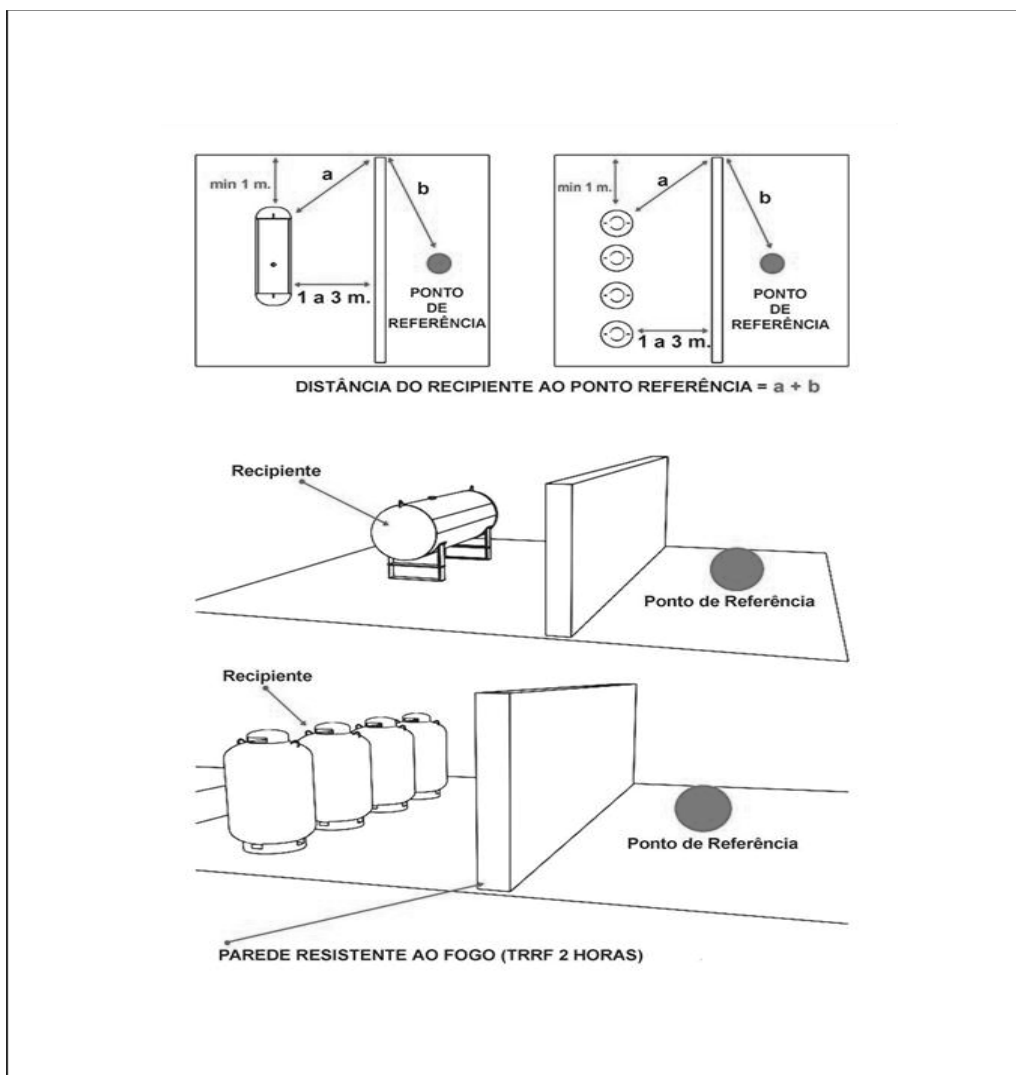
Figura 09: Exemplo de interposição de parede corta-fogo
