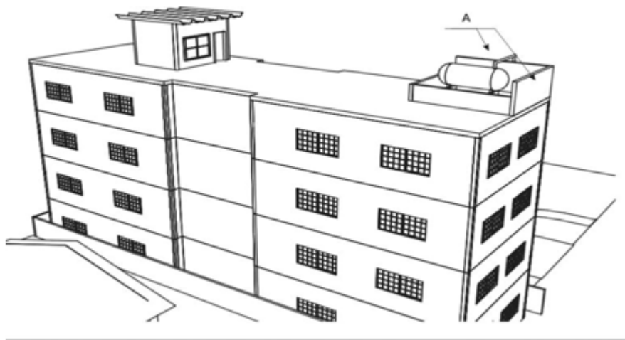
Figura 10b: Instalação de recipientes em teto e lajes de cobertura de edificações Nota: A - Paredes resistentes ao fogo
